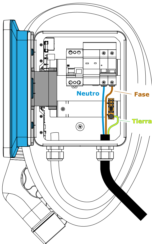
Diagrama modelo PRO
