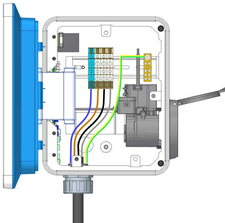
Diagrama modelo PLUG
